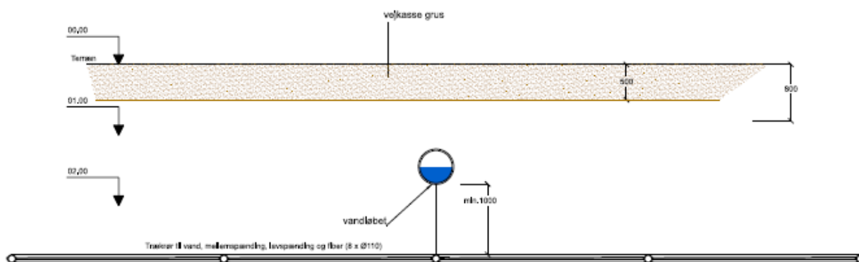
Kort 2. Snit med ledningsplacering ved krydsning af rørlagt del af Kærums å.
