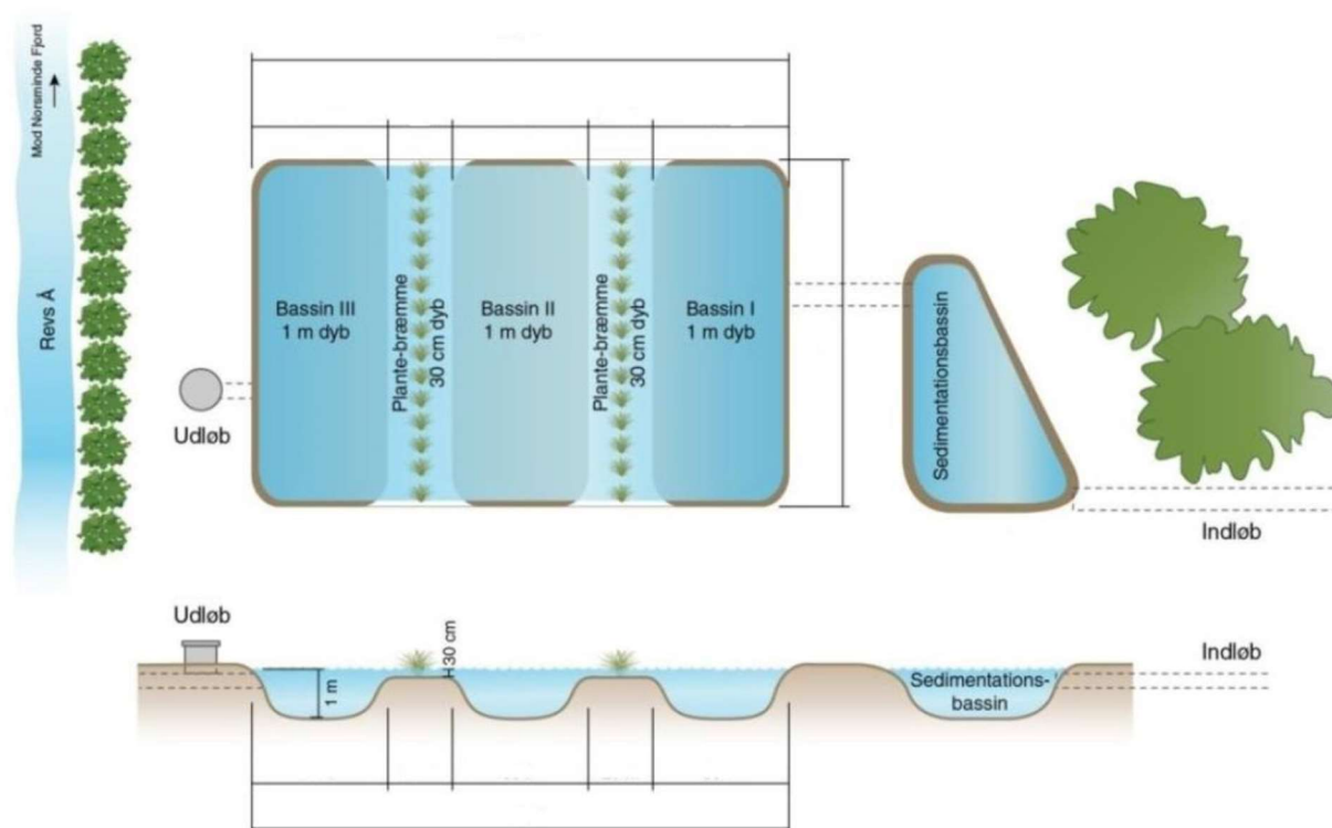
Fig. 2. Efter principskitse af design af minivåd område (Kjærgaard, C. & Hoffmann, C.C. 2013).
