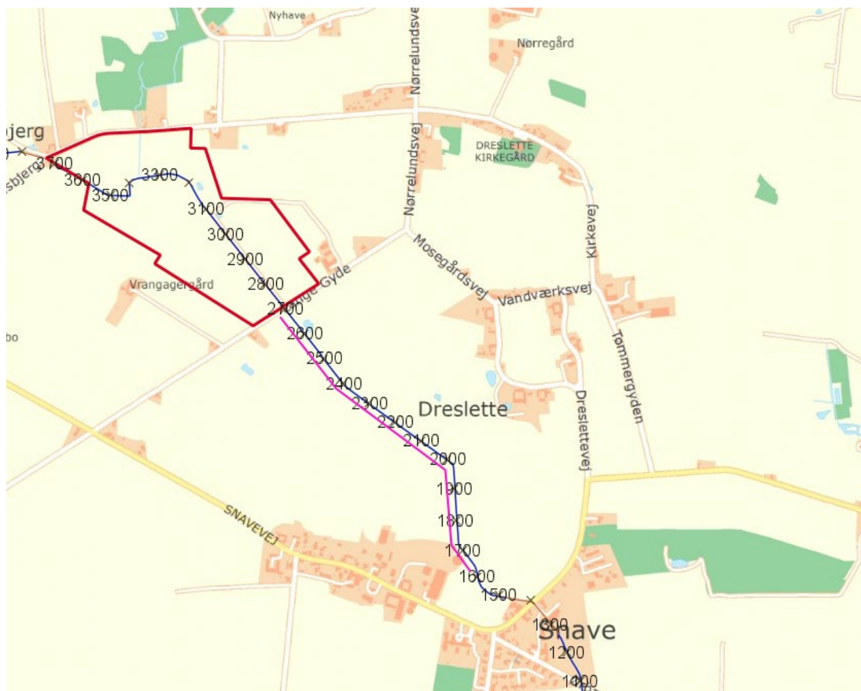
Figur 1: Vådområdeprojektet er markeret med rød signatur. Regulering opstrøms er markeret med lilla signatur. Vandløbets stationering er vist med sort skrift.
