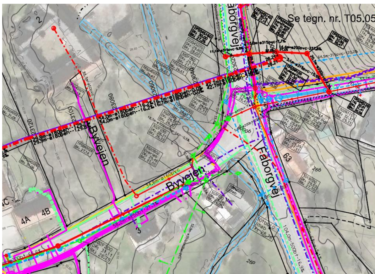
Kort. 1+2. Krydsning af Haarby Å omkring st. 10.705 ved Byvejen 2 i Køng/Gummerup
